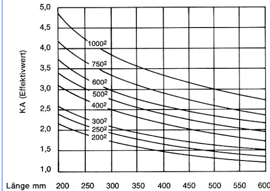
Belastungstabelle für luftgekühlte Schweißkabel (Richtwerte unverbindlich)
