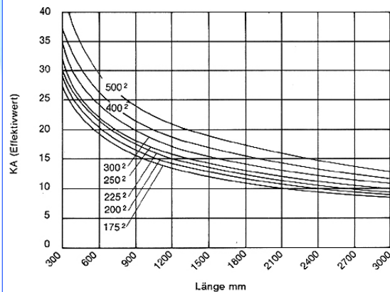
Belastungstabelle für wassergekühlte Schweißkabel (Richtwerte unverbindlich)
