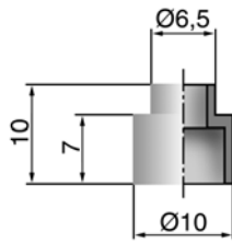
for M4 XE0.B04.000-01
