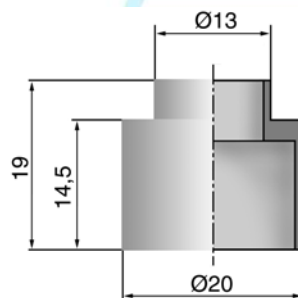
for M10 XE0.B10.000-01
