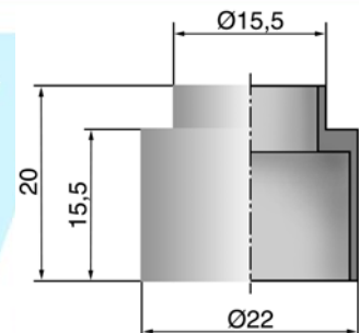
for M12 XE0.B12.000-01
