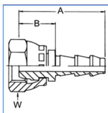
Dichtkopf für 60°-90° Konus
