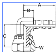
Dichtkopf für 60°-90° Konus, 90° Winkelstück
