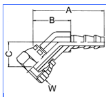
Dichtkopf für 60°-90° Konus, 45° Winkelstück
