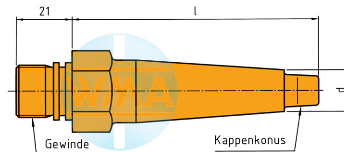
Einschraubkappenhalter C
