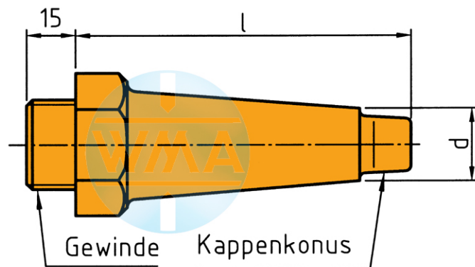
Einschraubkappenhalter B
