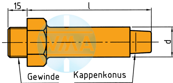
Einschraubkappenhalter A
