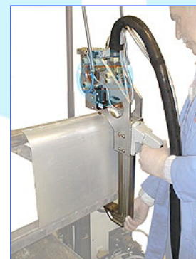
Spezialzange
